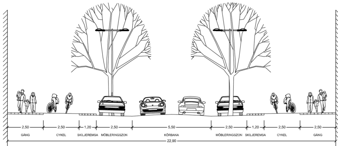
LOKALGATA DIM. FÖR LOKALT ENKELRIKTADE CYKELSTRÅK
